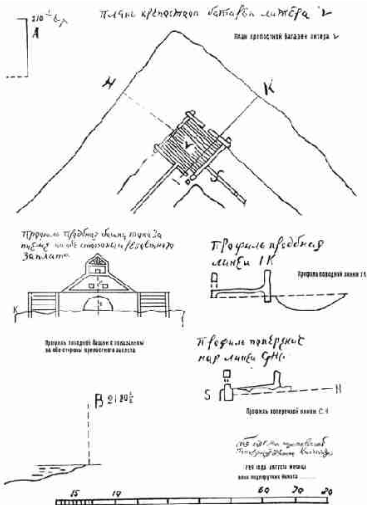
Рис. 7: Инженерный разрез бастионов Табынской крепости 1736 г.
